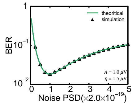
図2 BER 特性。
